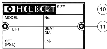
DETALLE -B- (PLACA DE IDENTIFICACIÓN)
