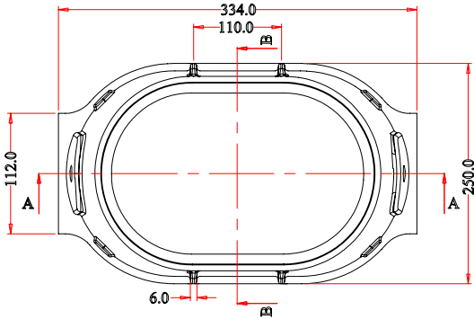
VISTA ARRIBA
