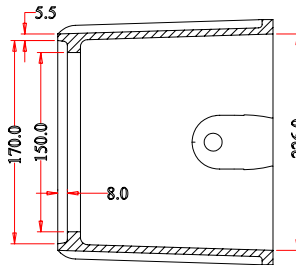
SECCION B-B
