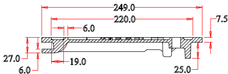
SECCION A-A
