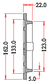
SECCION B-B
