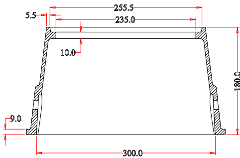
SECCION A-A
